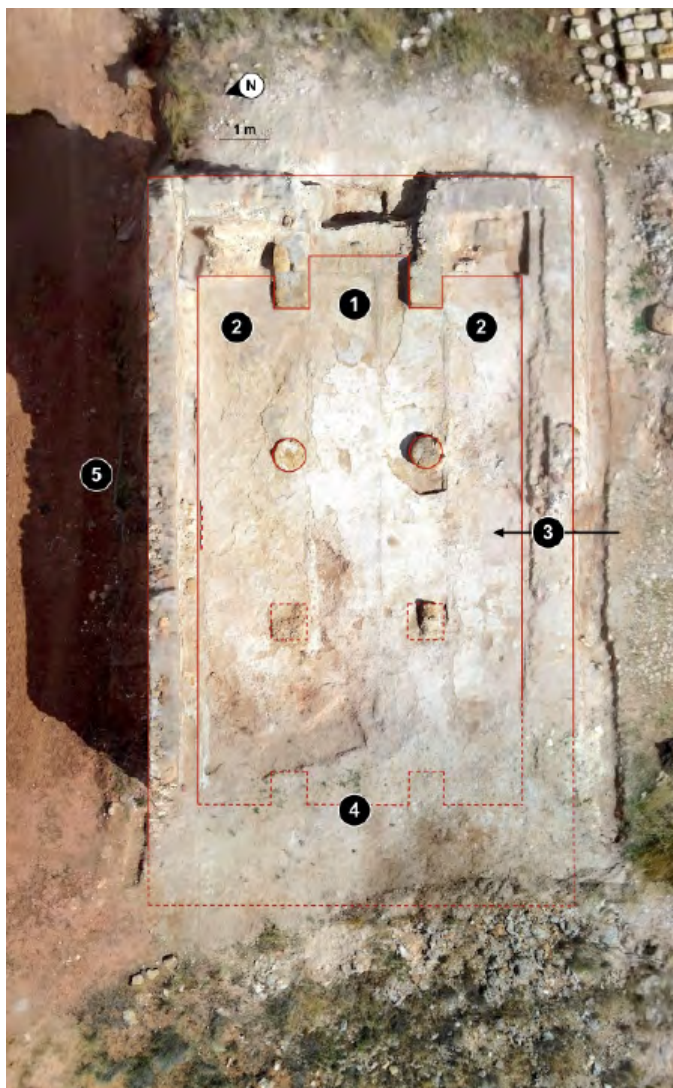
Fig. 5ª: Planta de la 1ª fase sobre la fotogrametría aérea del edificio: capilla mayor y nave central (1), capillas y naves laterales de la cabecera (2), puerta meridional (3), pies con posibles estructuras asociadas (4) y cementerio (5).
